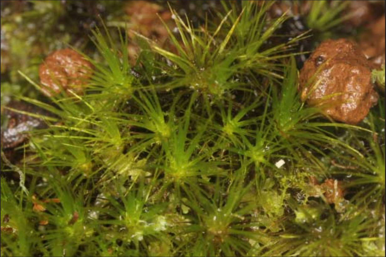
Campylopus laxitextus
